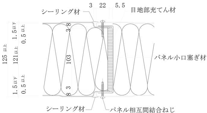
ジョイント部 断面詳細図
