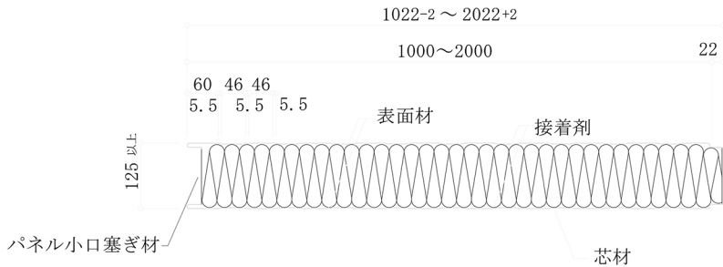
パネル単体断面詳細図
